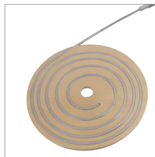
ploché topné těleso s výkonovým rozložením
